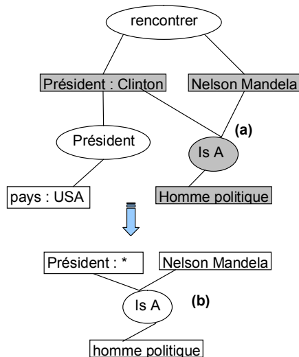
Figure 8: opérations de projection des GCs.
