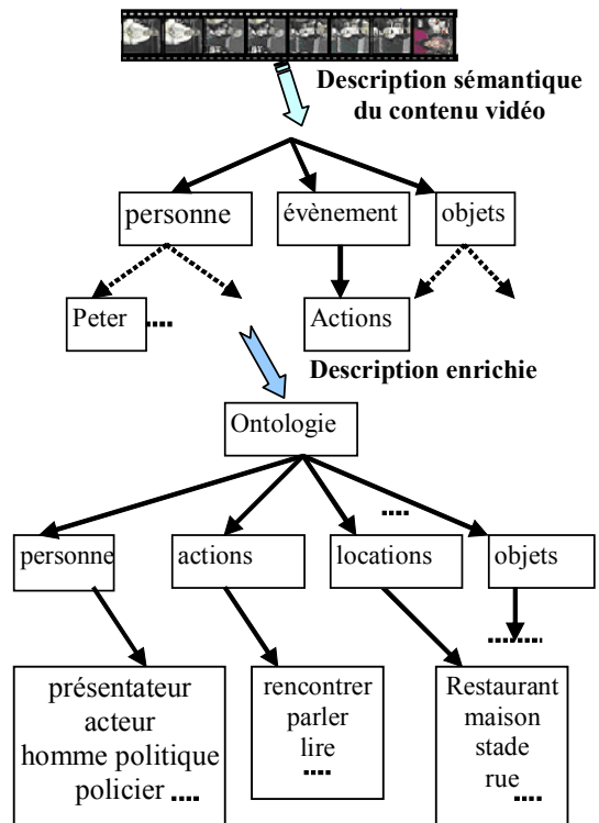
Figure 6: architecture pour la description du contenu sémantique
